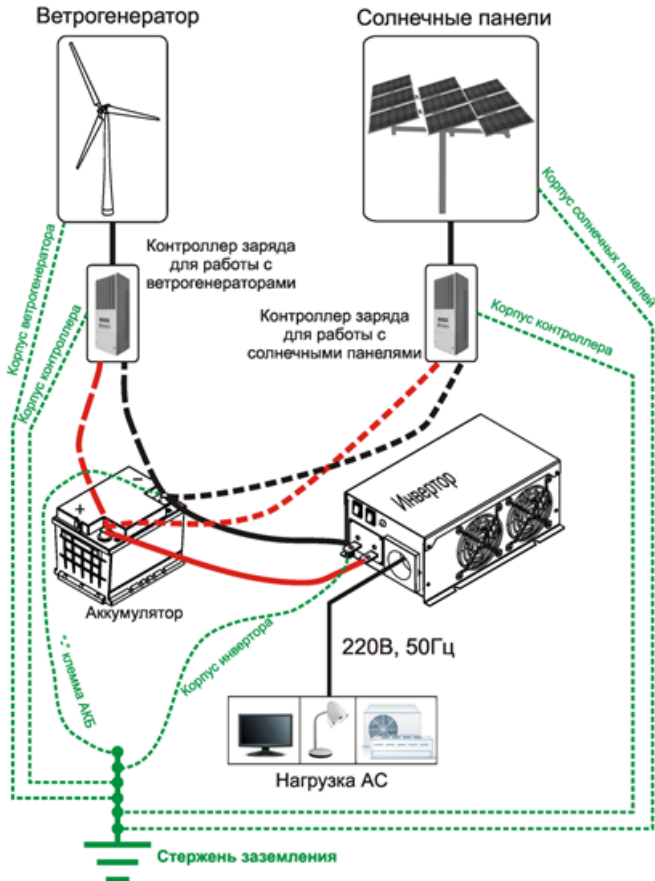
Рисунок 4 – Схема подключения инверторов серии СибВатт к системам альтернативной энергетики
